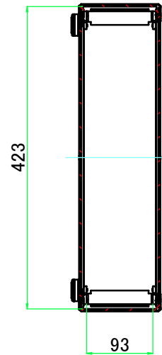
B-B ( 1 : 7.5 )
