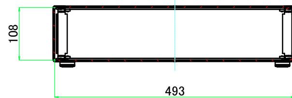
A-A ( 1 : 7.5 )
